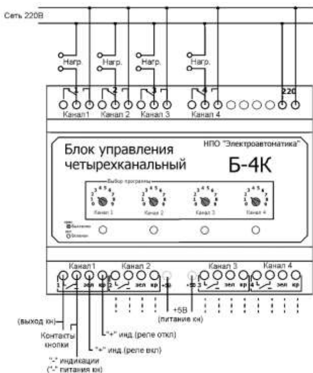
Рис. 2 Подключение устройства
