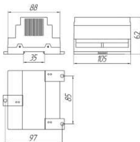
Рис. 1 Габаритные и установочные размеры
