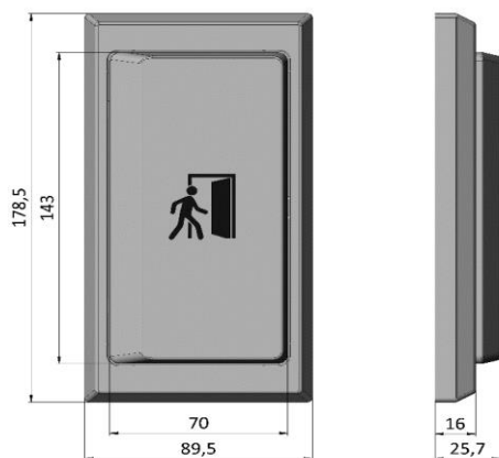
Рис. 1. Габаритные размеры
